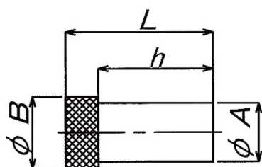
外観寸法図
