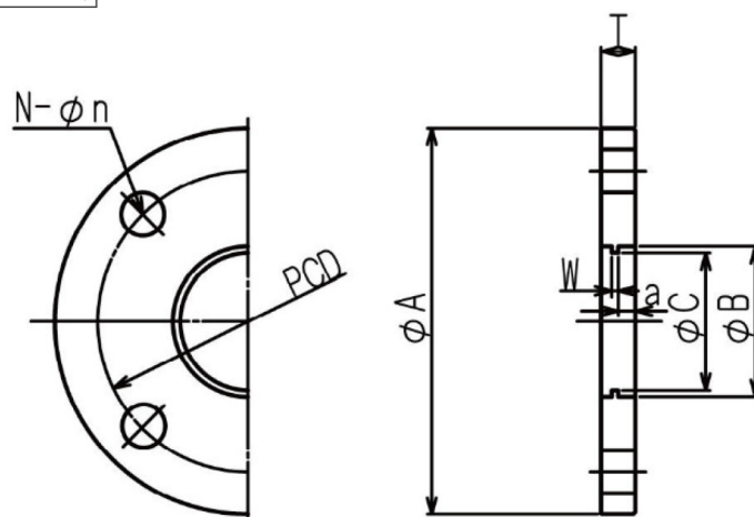
外観寸法図
