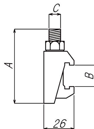
外観寸法図
