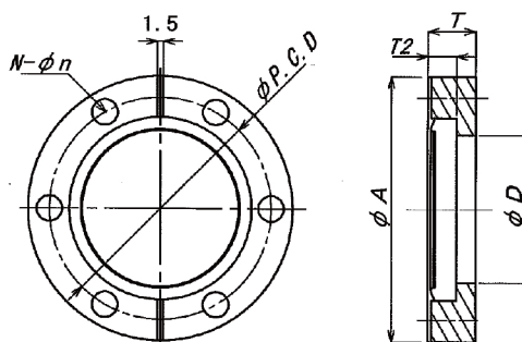
外観寸法図
