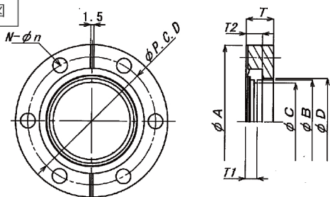
外観寸法図
