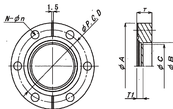
外観寸法図
