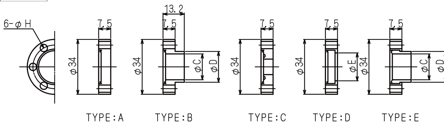
外観寸法図
