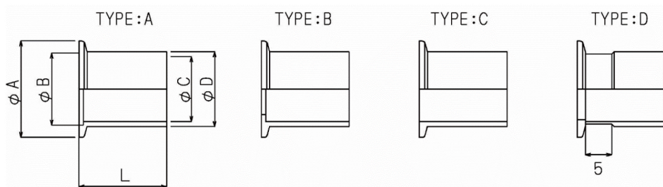
外観寸法図
