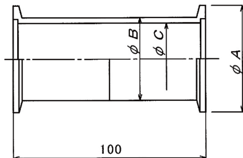
外観寸法図
