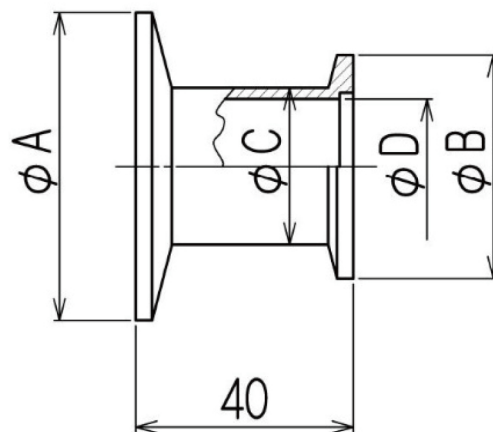
外観寸法図
