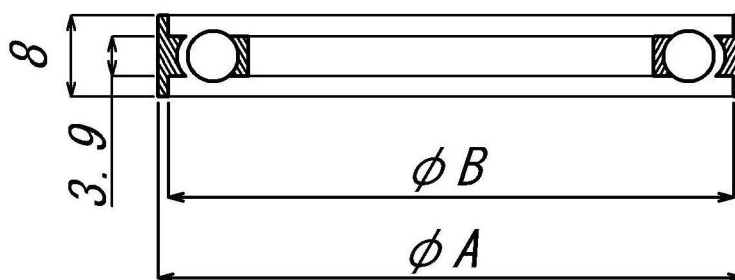
外観寸法図
