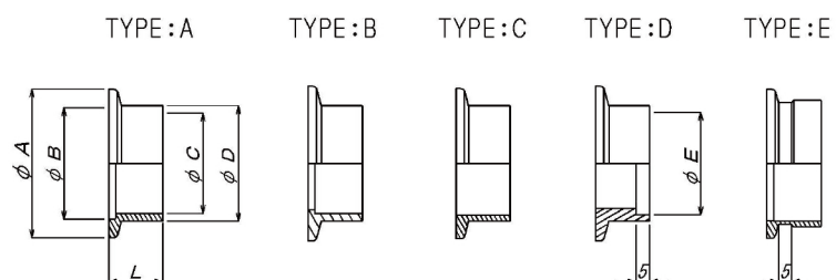
外観寸法図
